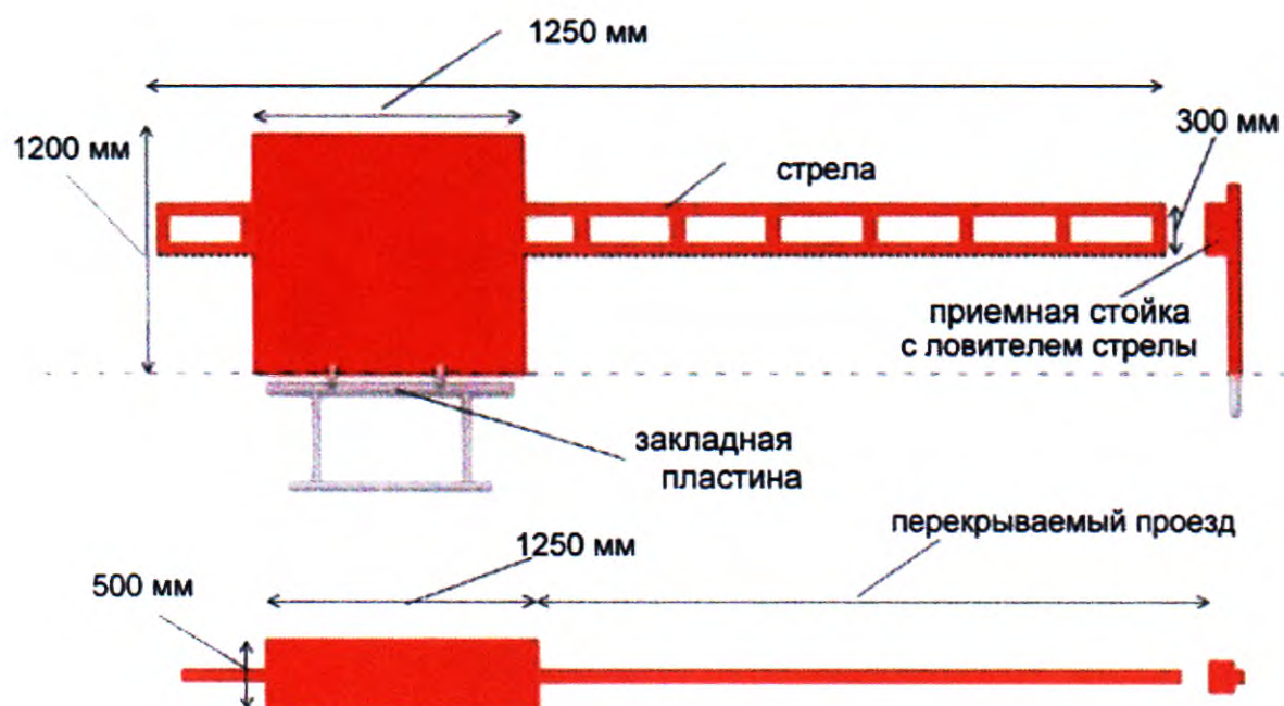
Рис. 2. Габаритные размеры
